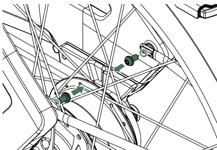
Figure 4 - Desserrer les boulons des béquilles de garde-boue.
