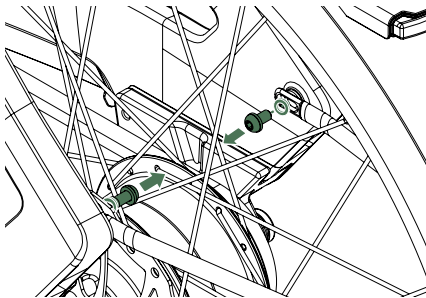
Figuur 4 - Spatbordstang bouten loshalen.
