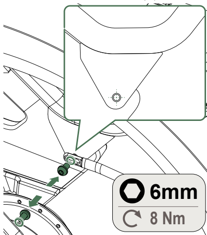
Figuur 6 - Achterste montagepunt uitlijnen.
