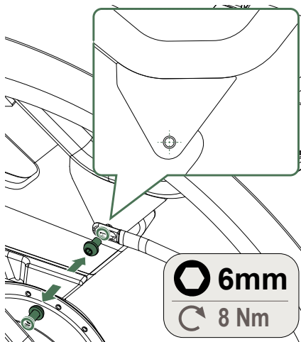
Figure 6 - Alignement du trou de montage arrière.
