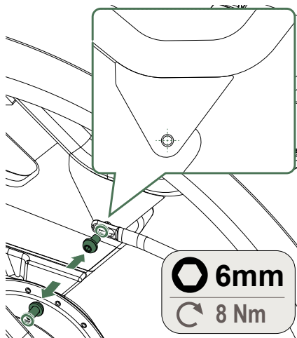
Abbildung 6 - Ausrichtung des hinteren Montagepunkts.
