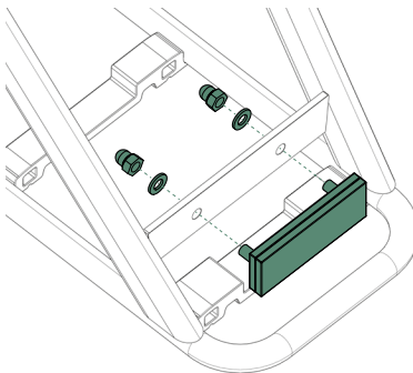
Abbildung 3 - Reflektor montieren.
