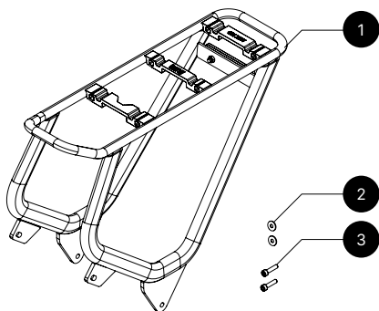
Figure 1 - Jeu de pièces.
