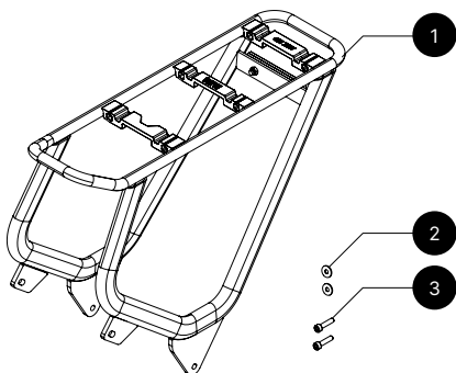
Figuur 1 - Onderdelen set.
