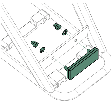
Figure 3 - Monter le réflecteur
