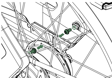
Abbildung 4 - Demontage der Schutzblechhalterung.
