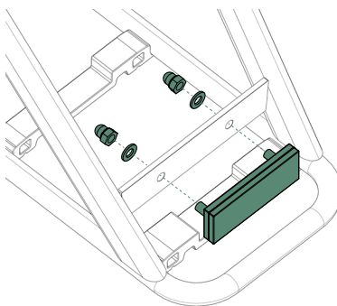
Figuur 3 - Reflector monteren.
