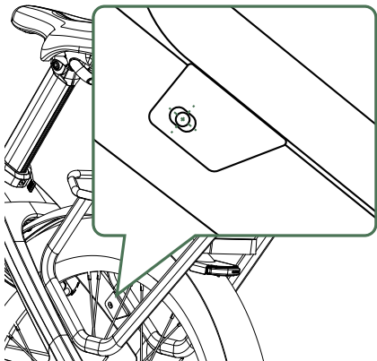
Figuur 5 - Voorste montagegat centreren.
