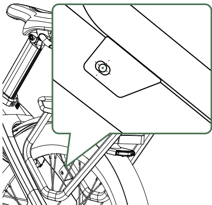
Figure 5 - Centrage du trou de montage avant.
