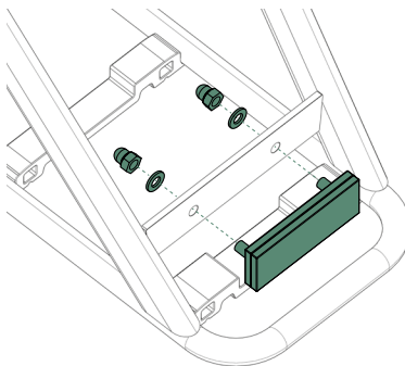
Figuur 3 - Reflector monteren.
